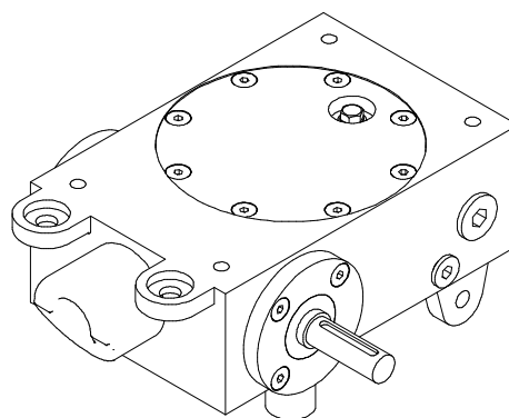
Caixa redutora completa
