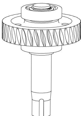
Roda de coroa completa
